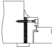
Joonis 2. Ukselengi ja ehitusavavaheline montaaživahe täidetakse tulekindla polüuretaanvahuga.
