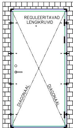
Joonis 1. Ukselengi fikseerimine ehitusavasasse. Vältimaks lengide väändumist ja tihendamaks püstlengide ja ülalpuu pragusid, tuleb paariskillud või tugiklotsid asetada ka ala- ja ülaurkadesse.
